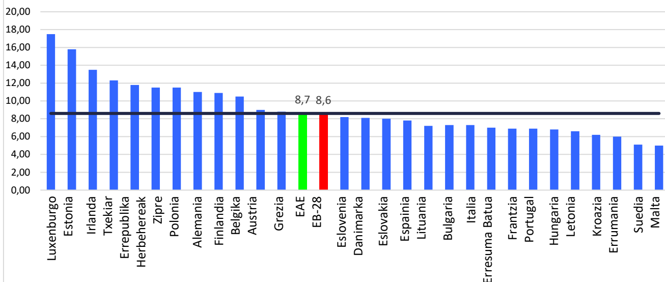
GRAFIKOA V.2.1. CO 2 -REN EMISIO RATIOAK EUSKADIKO ETA EB-28KO ESTATUETAKO BIZTANLE BAKOITZEKO (2018*)
