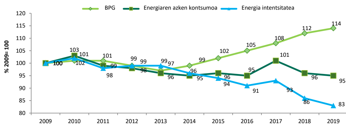
GRAFIKOA II.5.5. ENERGIA INTENSITATEAREN BILAKAERA
