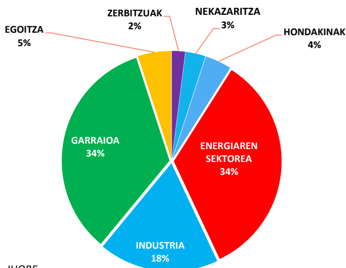
V.2.2. GRAFIKOA. BEG-EN EMISIO ZUZENAK EAE-KO SEKTOREEN ARABERA 2018-AN
